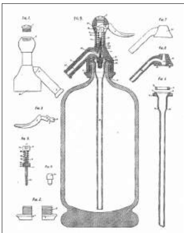
Corte en sección vertical de un envase de sifón, incluido en un catálogo de los talleres A. Vázquez del Saz, Madrid, 1914 (Archivo de Ángel Camacho)
