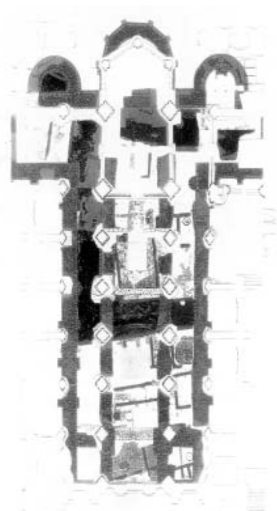
Fig. 3. Planta de la catedral de Pamplona. Después de las excavaciones de 1990
