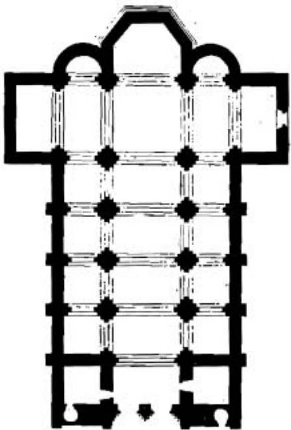
Fig. 2. Planta de la Catedral de Pamplona. Según Vicente Galbete Martinicorena
