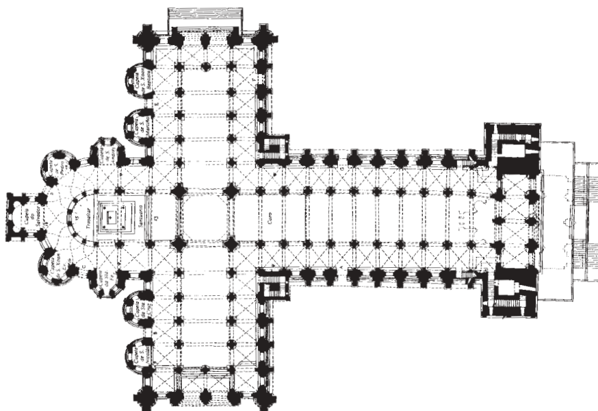
Fig. 4. Planta de la catedral de Santiago. Según Jhon Kenneth Conant
