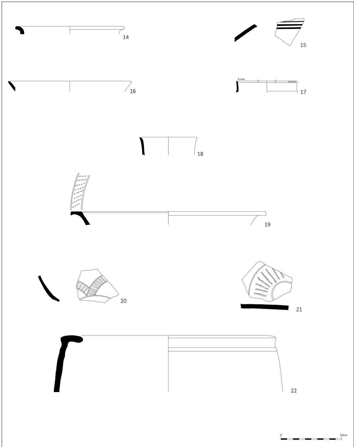
Figura 7. Segundo lote de materiales cerámicos estudiados.
