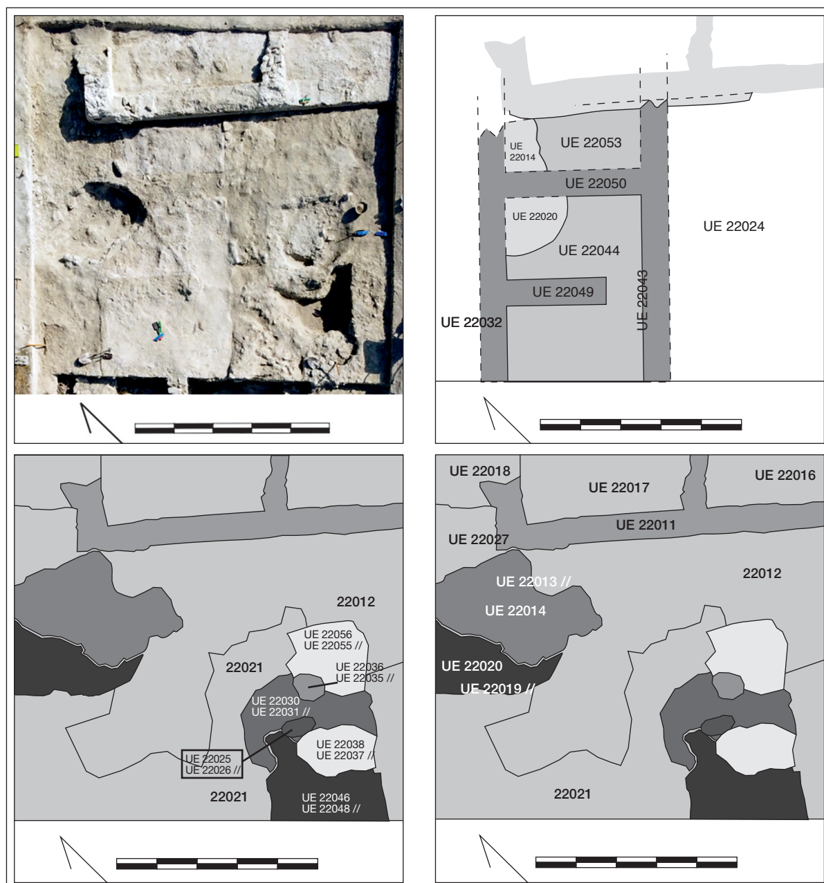
Figura 1. Vista cenital y localización de las diferentes unidades estratigráficas.
