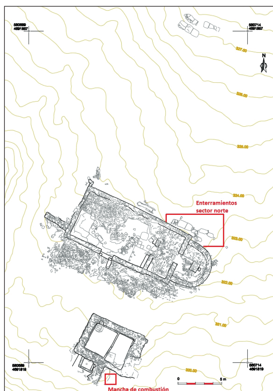
Figura 1. Planta general del complejo eclesiástico de Resa, con indicación de las áreas excavadas en 2025.
